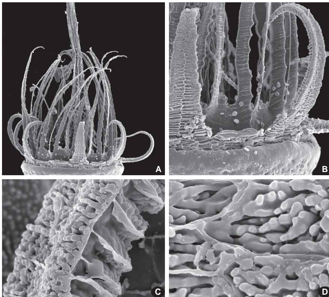
Рис. 493. Climacium dendroides (Hedw.) Web. et Mohr: А – перистом и длинно выбегающая колонка, \times 36 ; В – часть перистома: некоторые зубцы обломаны, что позволяет видеть расщепленные почти до основания сегменты эндостома на низкой базальной мембране без ресничек, \times 145 ; С – зубцы экзостома в средней части, вид сбоку, позволяющий видеть часто расположенные вентральные трабекулы, \times 1200 ; D – орнаментация зубца экзостома снаружи в нижней части, \times 2400 .
