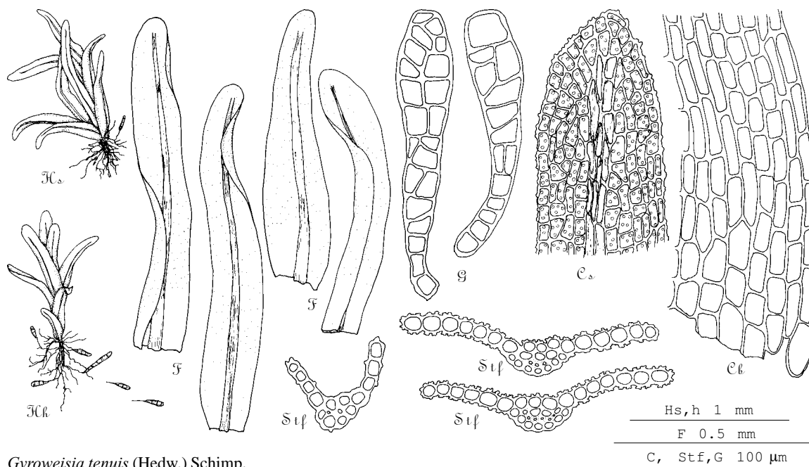
Gyroweisia tenuis (Hedw.) Schimp.
