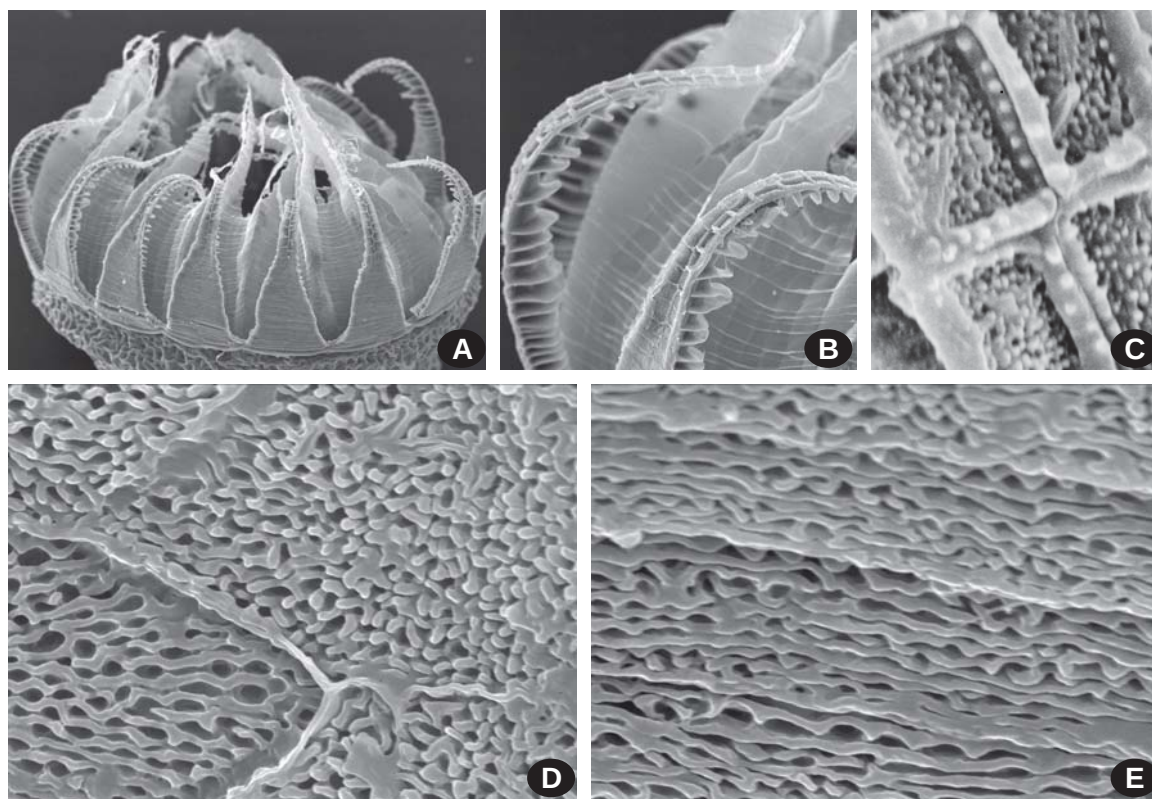
Рис. 189. Детали строения перистоста Hylocomium splendens : А – перистом, \times 60 ; В – зубцы экзостоста сбоку вверх, \times 165 ; С–Е – орнаментация зубцов экзостоста на дорсальной стороне в верхней (С, \times 1800 ), средней (D, \times 3000 ) и нижней (Е, \times 3300 ) частях.
